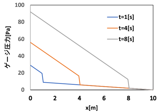
図 1 VOF 解析の圧力分布の時間発展
