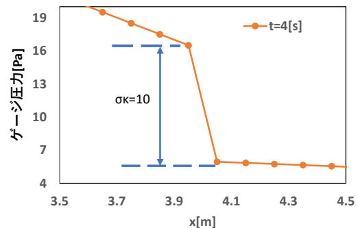
図 2 t=4[s] の界面近傍の圧力分布
