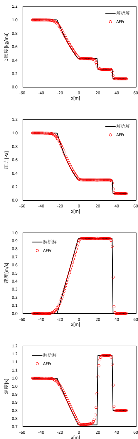
図 5 AFFr による 1 次元衝撃波管解析
