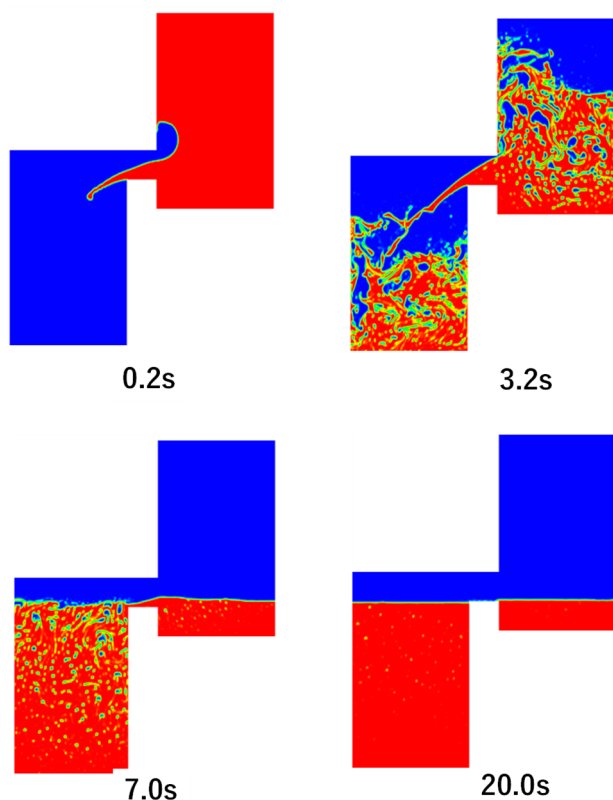
図 3 AFFr による 2 次元タンク放水解析
