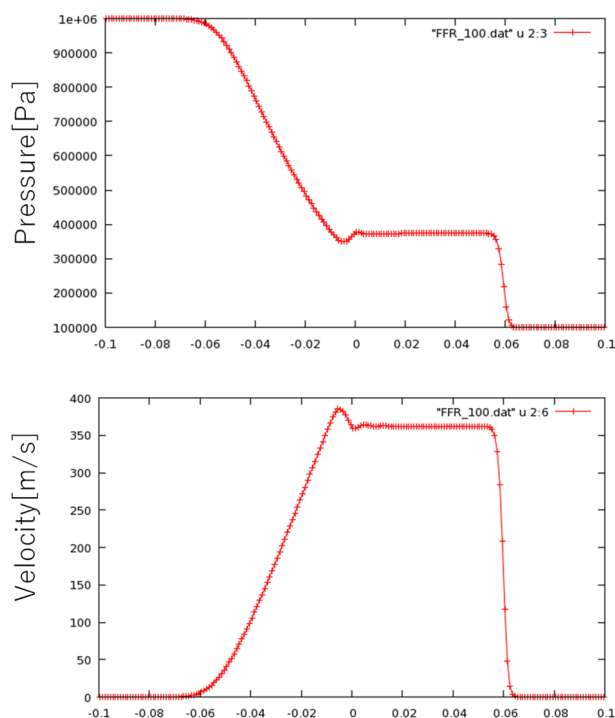
図 4 AFFr SIMPLE 法による衝撃波解析 上: 圧力、下: 速度
